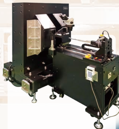
FMR測定装置
